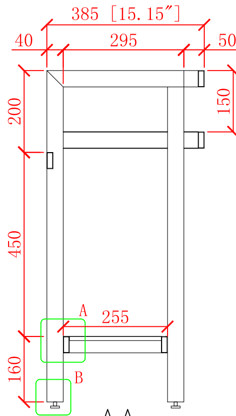
A-A 1:1
